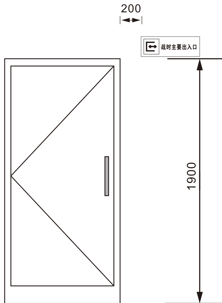
口部标识牌安装示例
