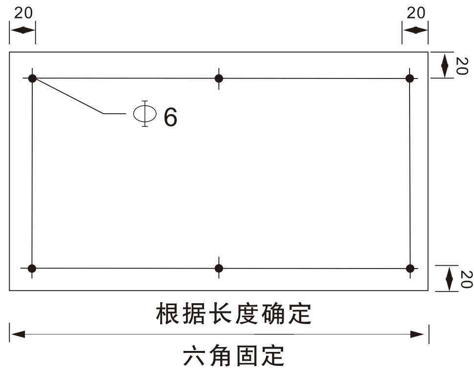
图2 六孔固定安装示意图
